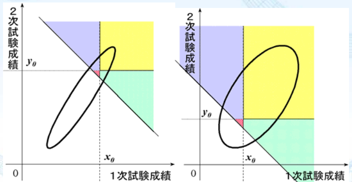
図7 相関による影響
