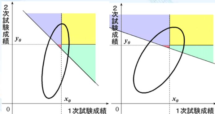
図9 分散の違いによる影響
